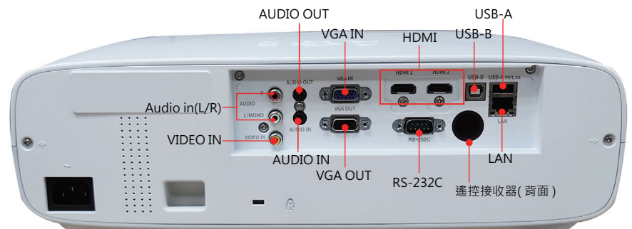
輸 入 端 子
